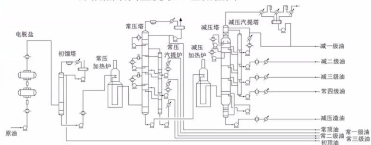
原油蒸馏真空提取工艺流程图
